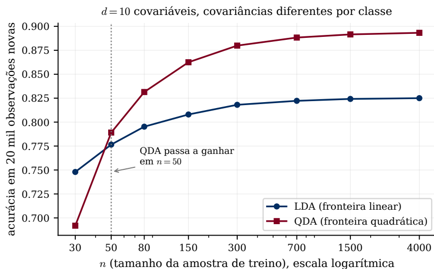
Figura 2: Acurácia dos dois métodos em função de n , com d = 10 covariáveis e covariâncias genuinamente diferentes por classe — ou seja, num cenário em que o QDA está certo e o LDA está errado . Ainda assim, com n = 30 o LDA ganha (0,748 contra 0,692): não há dados para estimar 110 parâmetros de covariância, e a variância do QDA supera o viés do LDA. A partir de n = 50 o jogo vira, e em n = 4000 o QDA abre sete pontos percentuais. Médias de 120 repetições, avaliadas em 20 000 observações novas.
